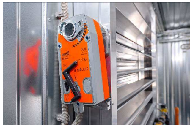
Внутри - автоматические клапаны притока-оттока воздуха с электроприводом Belimo 24/220 В
