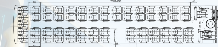
Планировка междугороднего автобуса Scania Higer A80 6x2*4
