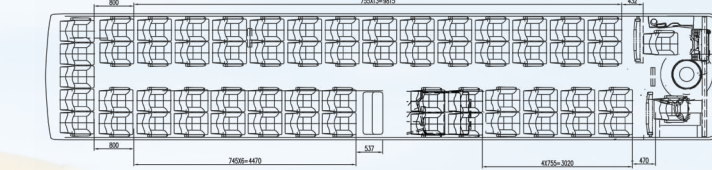
Планировка туристического автобуса Scania Higer A80 6x2*4
