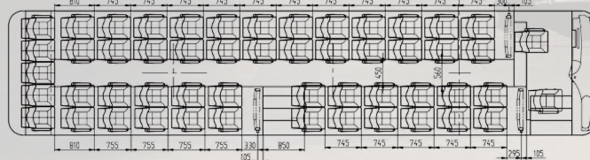
Планировка междугороднего автобуса Scania Higer A80 4x2
