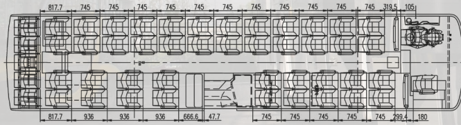
Планировка туристического автобуса Scania Higer A80 4x2
