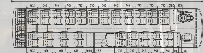
Планировка туристического автобуса Scania Higer A80 4x2
