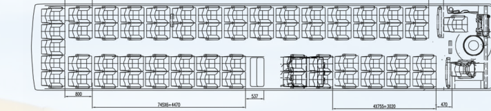
Планировка туристического автобуса Scania Higer A80 6x2*4
