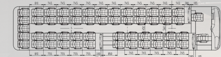
Планировка междугороднего автобуса Scania Higer A80 4x2
