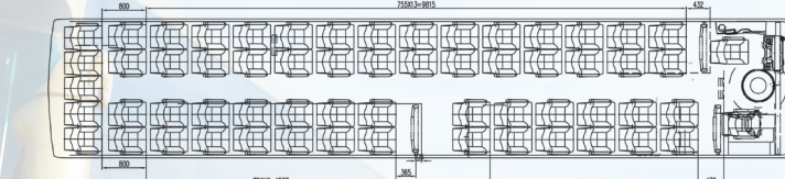
Планировка междугороднего автобуса Scania Higer A80 6x2*4
